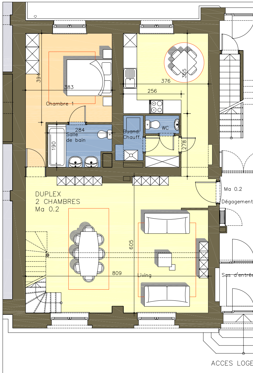
Rez-de-chaussée
